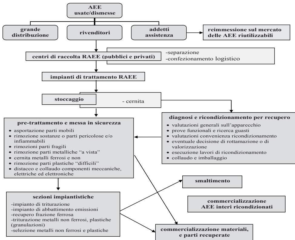
Figura 2: Schema di massima sulla gestione dei RAEE
